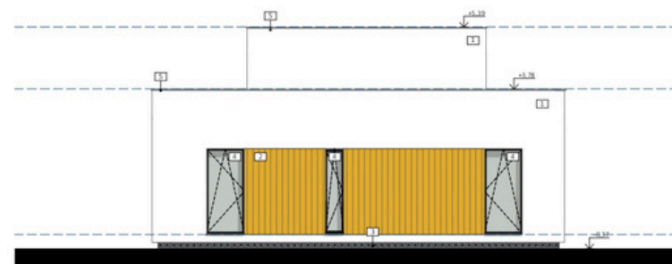
ELEVACJA BOCZNA_2
