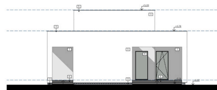
ELEVACJA BOCZNA_1
